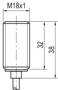
Габаритный чертеж
